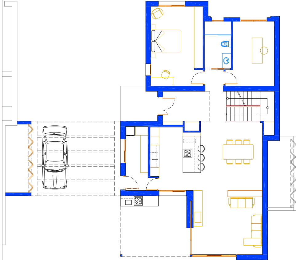
PLANTA BAJA
