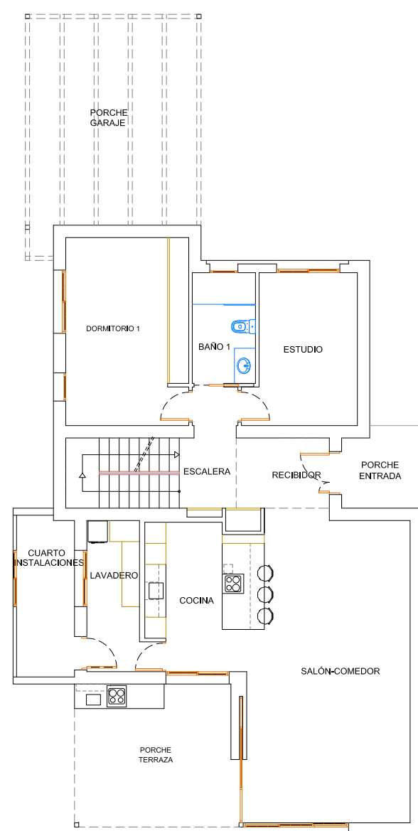
PLANTA BAJA
