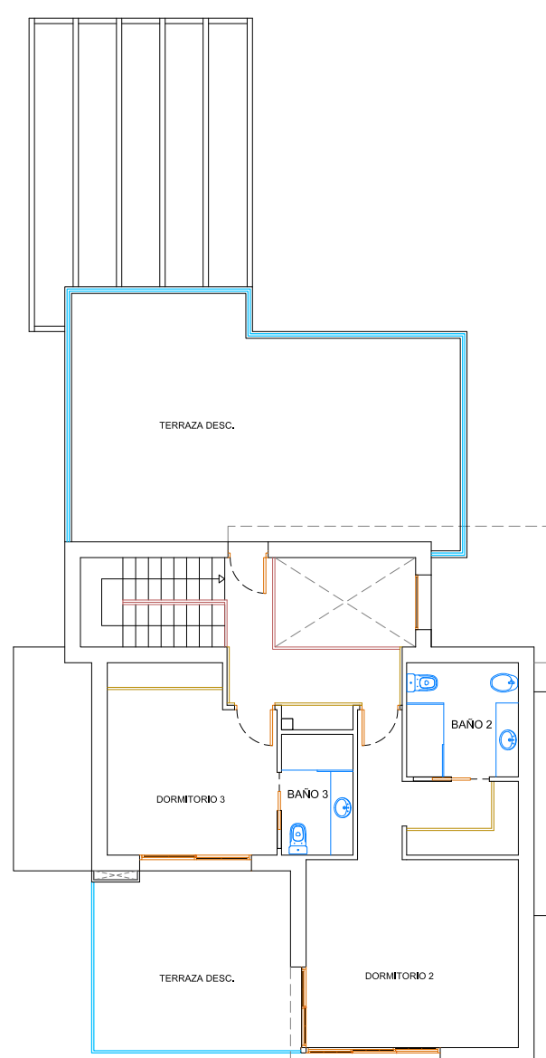
PLANTA PRIMERA
