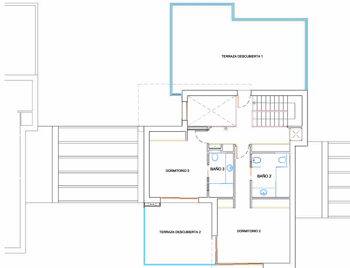
PLANTA PRIMERA
